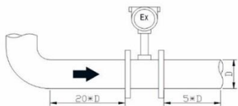
3. 1*90° 弯管
