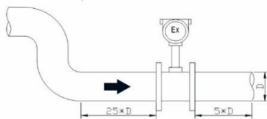
4. 在同一平面2*90° 弯管
