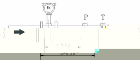
7. 涡街流量传感器同压力传感器和温度传感器组成测量系统时，其压力、温度测量点的位置图
